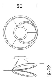
Kepler petite
